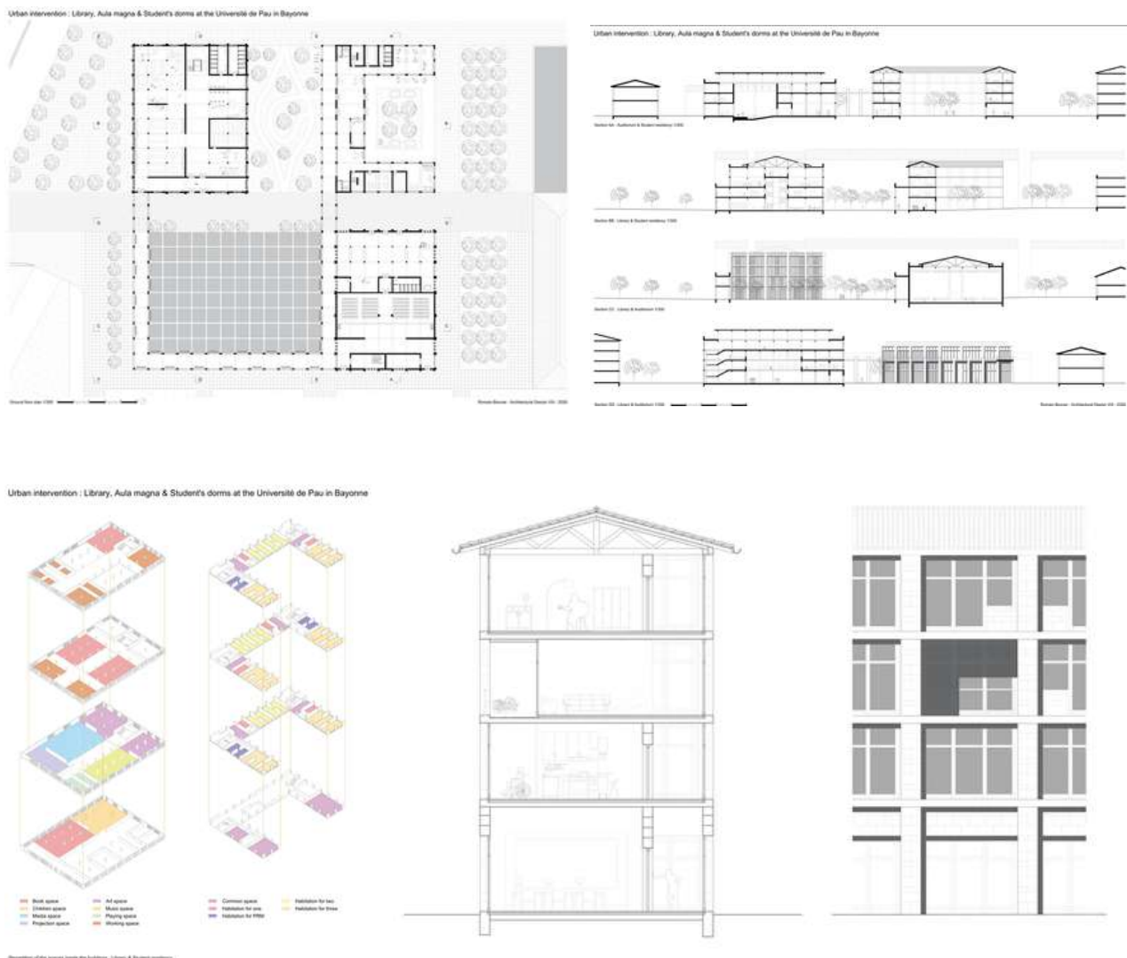
Plan RDC, coupes, façades, axono des espaces et détails 50 du projet
