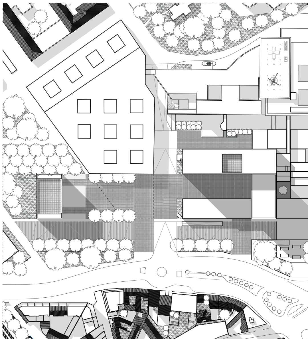
Plan de masse 1/500
