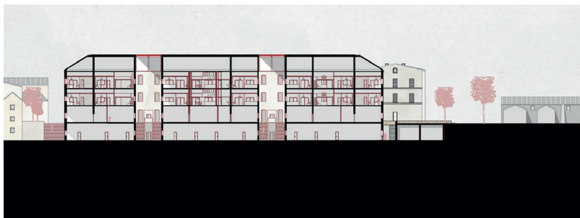
COUPE LONGITUDINALE CASERNE FRANCAISE
