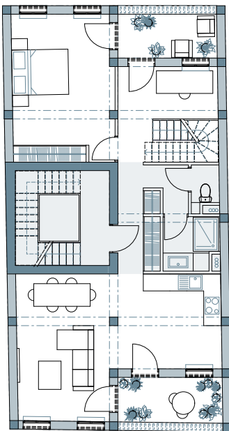
Plan de R+2, 1/50 Un T4 en duplex, premier niveau de 75 m 2 avec deux balcons de 5 m 2
