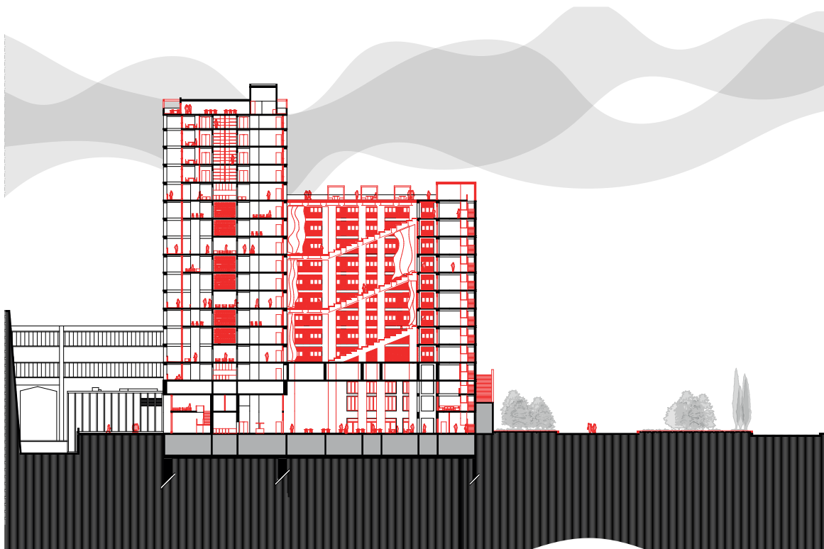
COUPE C2
