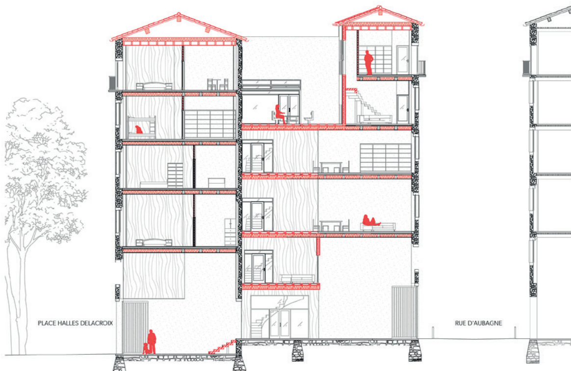
COUPE LONGITUDINALE
