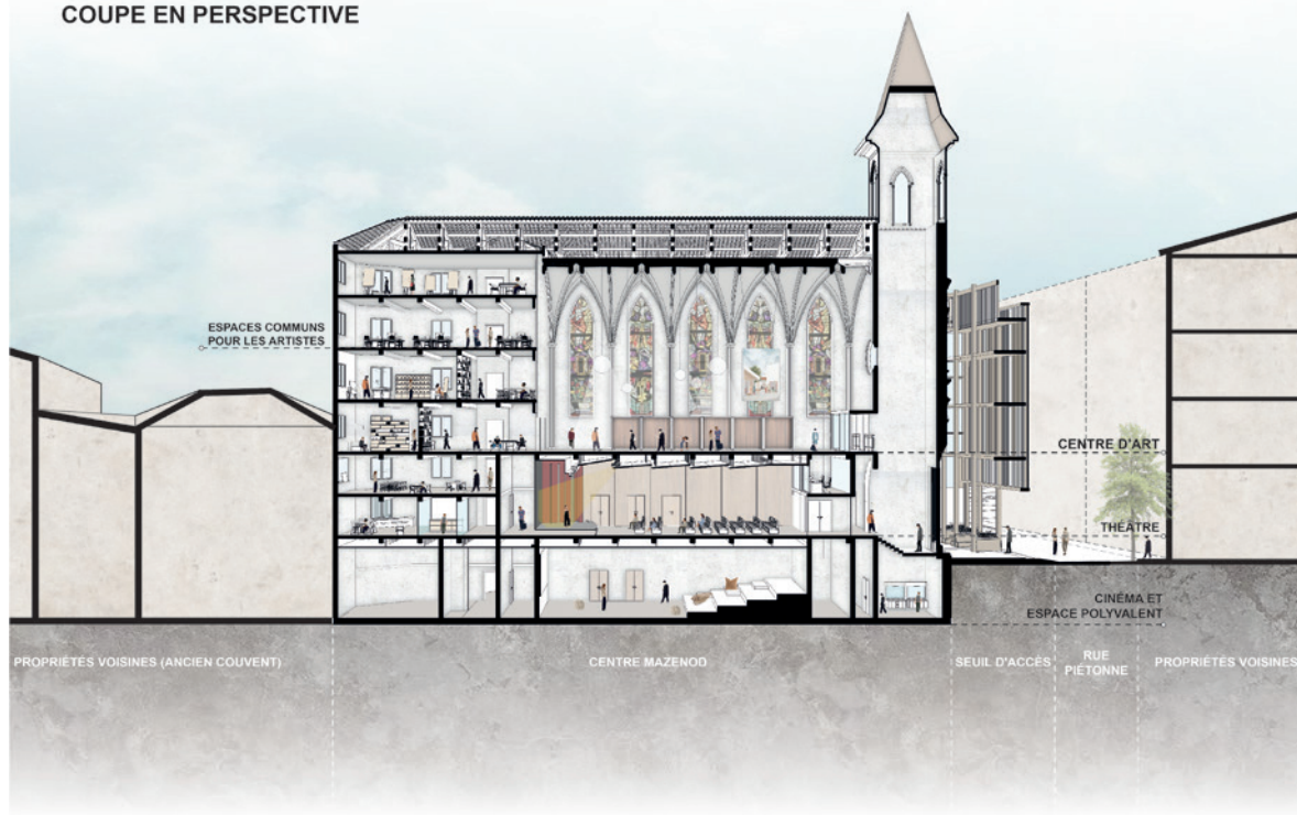
COUPE LONGITUDINALE
