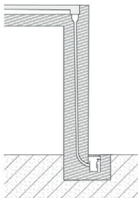
DÉTAIL BLOC 1/20
