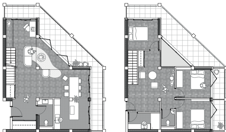
Plan logement en duplex - 1/20e
