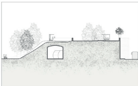
Coupe sur l'axe de bus supérieur
