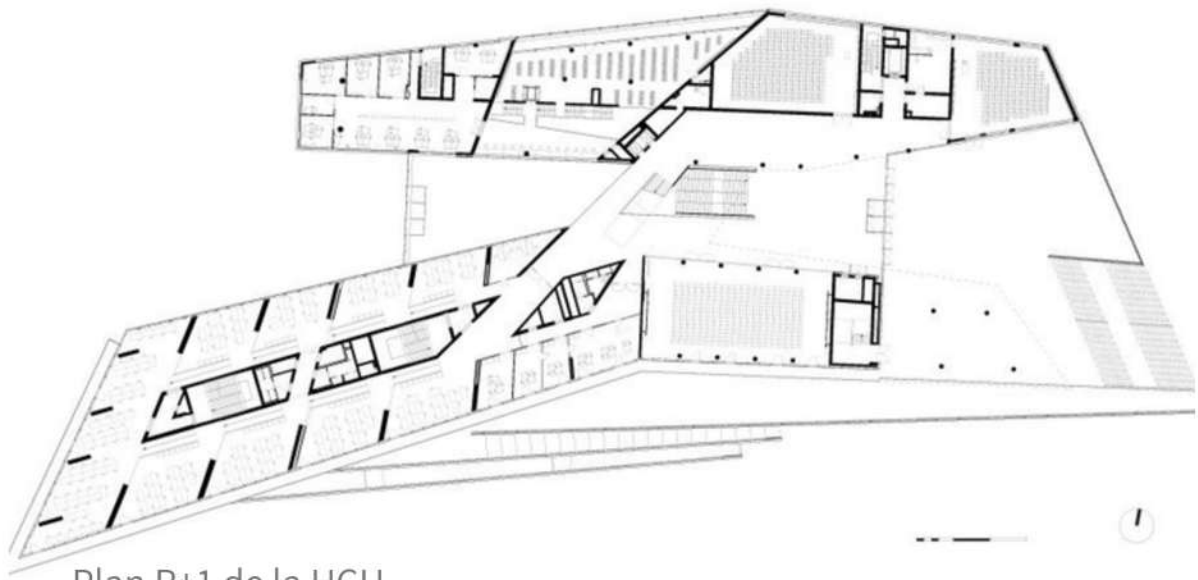
Plan R+1 de la HCU
