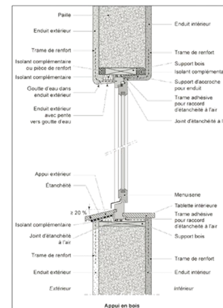
Source : extraits des Règles Professionnelles de Construction en Paille - 2 e édition. Le Moniteur, 2014, p.84-p.100
